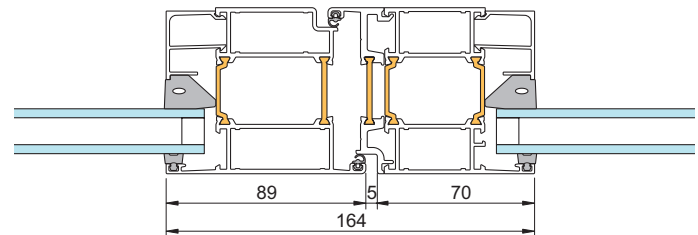
7 - Dør med sidelys. Smalprofil med utskiftbart anslag
