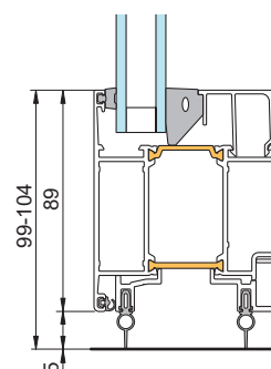
3 - Dør med slepetetting
