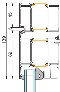
4 - OK dør med karm
