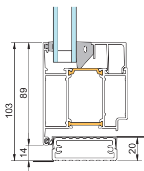
3 - Dør med anlagstetting mot rustfri, uisolert terskel
