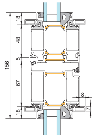
8 - OK dør med overlys
