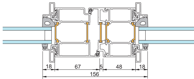
7 - Dør med sidelys
