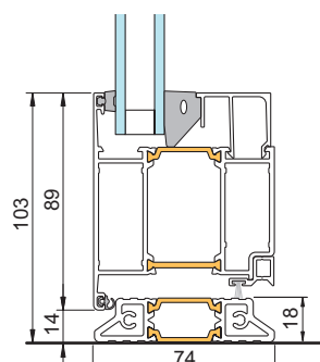
3 - Dør med anlagstetting mot faset terskel
